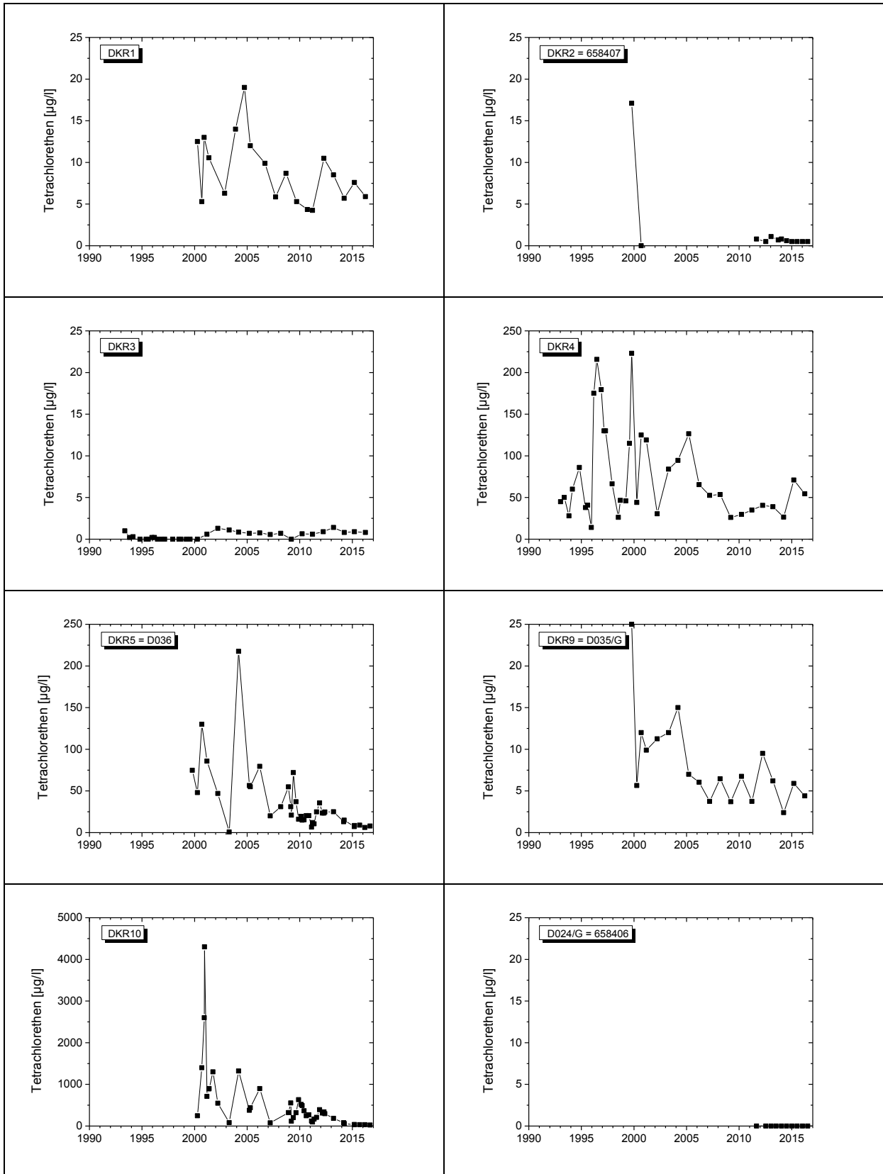
Zeitliche Entwicklung der Tetrachlorethenkonzentration in acht Grundwassermessstellen
